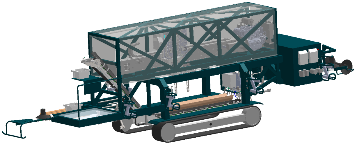
Impressie 1-rijige zelftrekkende Sparter
